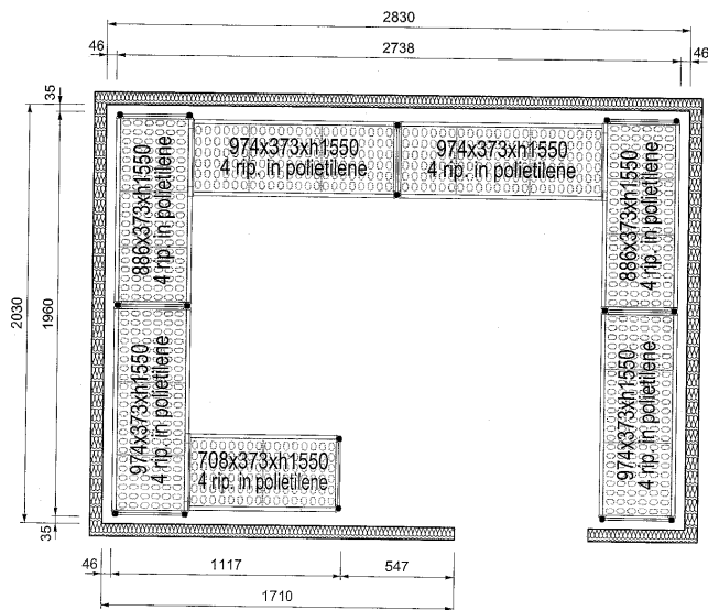
Boven aanzicht
